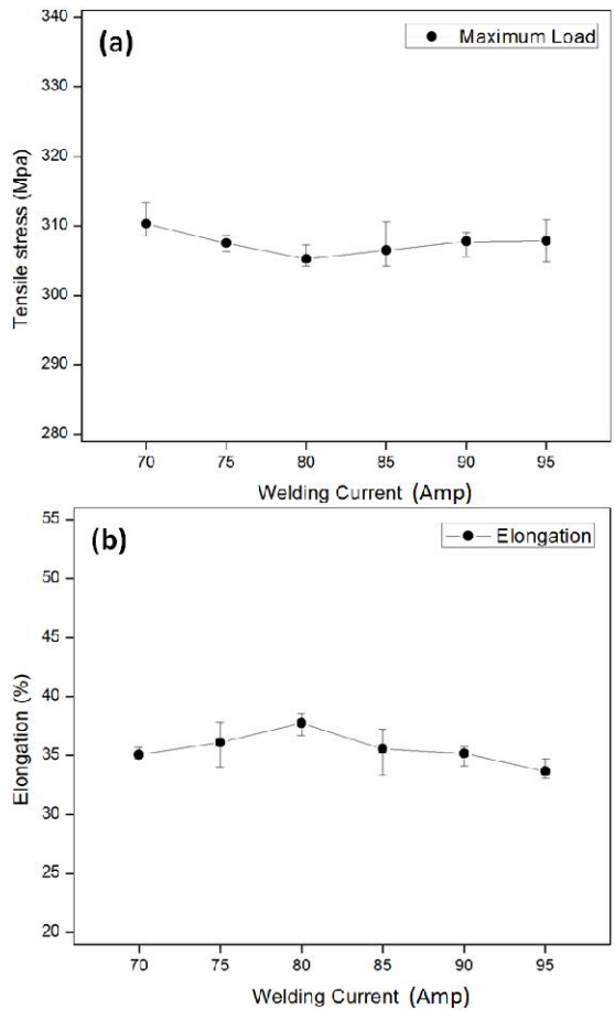
รูปที่ 4 (a) กราฟแสดงความแข็งแรงทานแรงดึงสูงสุดของชิ้นงานในแต่ละกระแสเชื่อม และ (b) กราฟแสดงเปอร์เซ็นต์การยืดตัวของชิ้นงานในแต่ละกระแสเชื่อม
