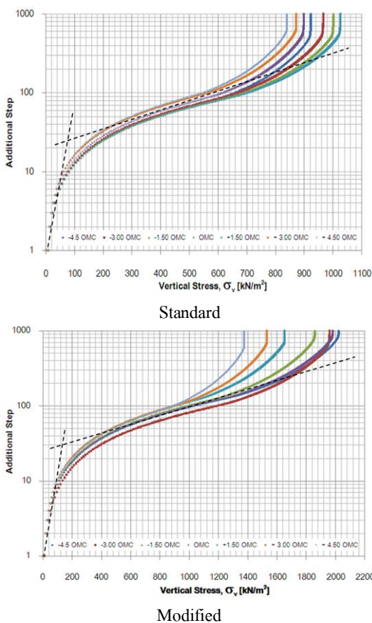
รูปที่ 12 ผลการวิเคราะห์หาค่าหน่วยแรงในมวลดินที่จุดวิกฤติภายใต้้น้ำหนักบรรทุก
