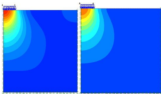
รูปที่ 10 การเคลื่อนตัวของมวลดินที่จุดวิบัติ
