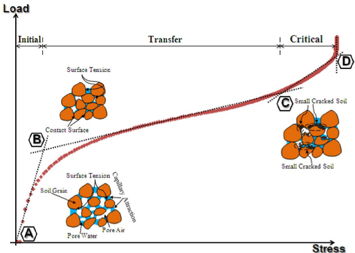
รูปที่ 13 กลไกการรับน้ำหนักของมวลดินลูกรังบดอัด
