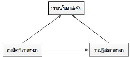
รูปที่ 24 ตัวแบบเส้นทางแสดงอิทธิพลของการป้องกันการเสพยาที่มีต่อการปฏิเสธยาที่มีการต่อต้านยาเสพติดเป็นตัวแปรคั่นกลาง
