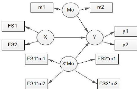
รูปที่ 13 การวิเคราะห์ตัวแบบการกำกับกรณี second order model มีตัวแปรกำกับ ขั้นที่ 2
