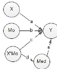
รูปที่ 30 ตัวแบบ mediated moderation model
