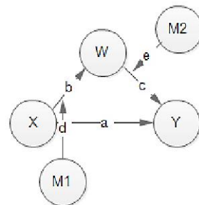
รูปที่ 16 ตัวแบบที่มีตัวแปรกำกับ 2 ตัว 2 เส้นทาง
