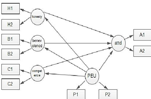
รูปที่ 9 ตัวอย่างวิธีวิเคราะห์ด้วย build up approach ขั้นที่ 1
