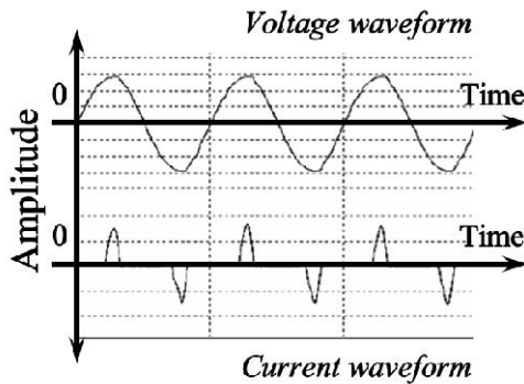
รูปที่ 3 รูปคลื่นของสวิทซ์ซิ่งเพาเวอร์ซัพพลาย [3]
