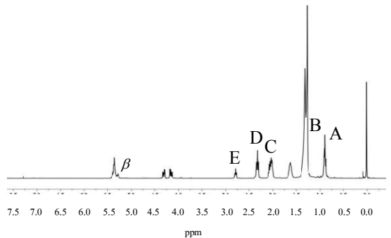
รูปที่ 2 แสดงสเปกตรัม 400 MHz 1 H NMR ของน้ำมันรำข้าวบิบเย็นจากลพบุรี (L-RBO12)
