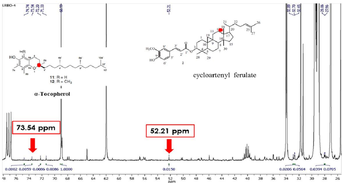
รูปที่ 5 แสดงสเปกตรัม 13 C NMR ของน้ำมันรำข้าวบีนเขินจากลพบุรี (L-RBO12)
