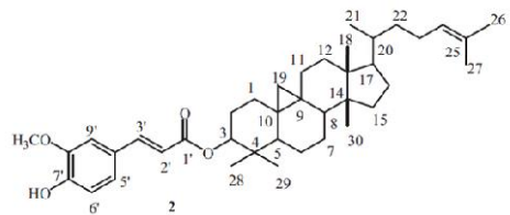
รูปที่ 1 แสดงโครงสร้างของสารประกอบออโรซินอล (cycloeucalenol cis -ferulate)
