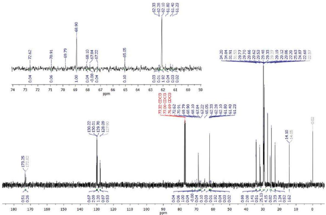
รูปที่ 3 แสดงสเปกตรัม 13 C NMR ของน้ำมันรำข้าวบิบบิ้นจากโยธร (Y-RBO1)
