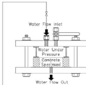
รูปที่ 4 การทดสอบหาค่าการซึมของน้ำผ่านคอนกรีต โดยอาศัยหลักการไหลของน้ำที่คงที่
