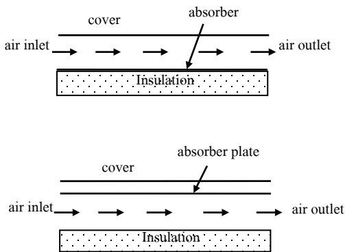
รูปที่ 4 ตัวเก็บรังสีแบบช่องทางเดียว (Single-pass air solar heater) (ดัดแปลงจาก [7])
